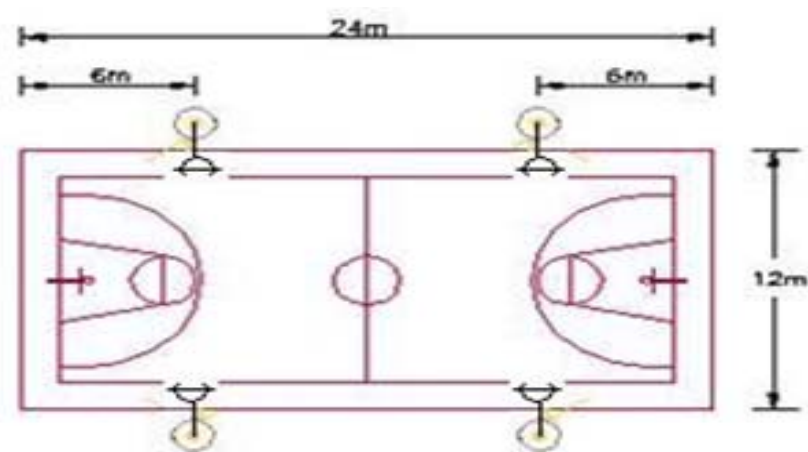
Figura 560.3.3 b. Cancha múltiple sencilla
