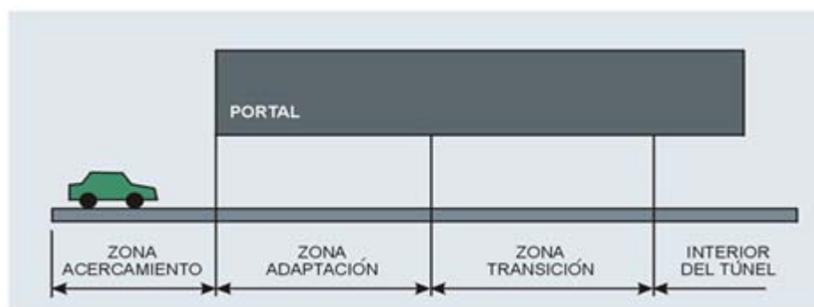
Figura 570 Zonas lumínicas de un túnel
