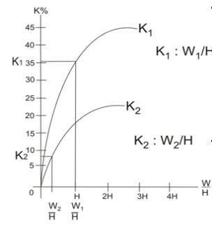
Figura 530.2.2 b. Curvas de coeficiente de Utilización
