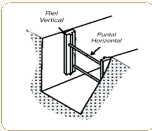
Figura 5 Apuntalamiento hidráulico
