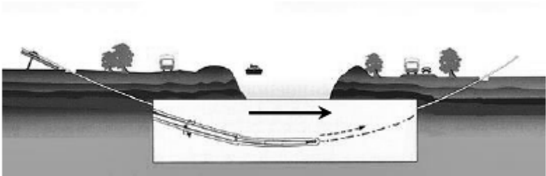
Perforación del paso del piloto a lo largo de la trayectoria planeada
